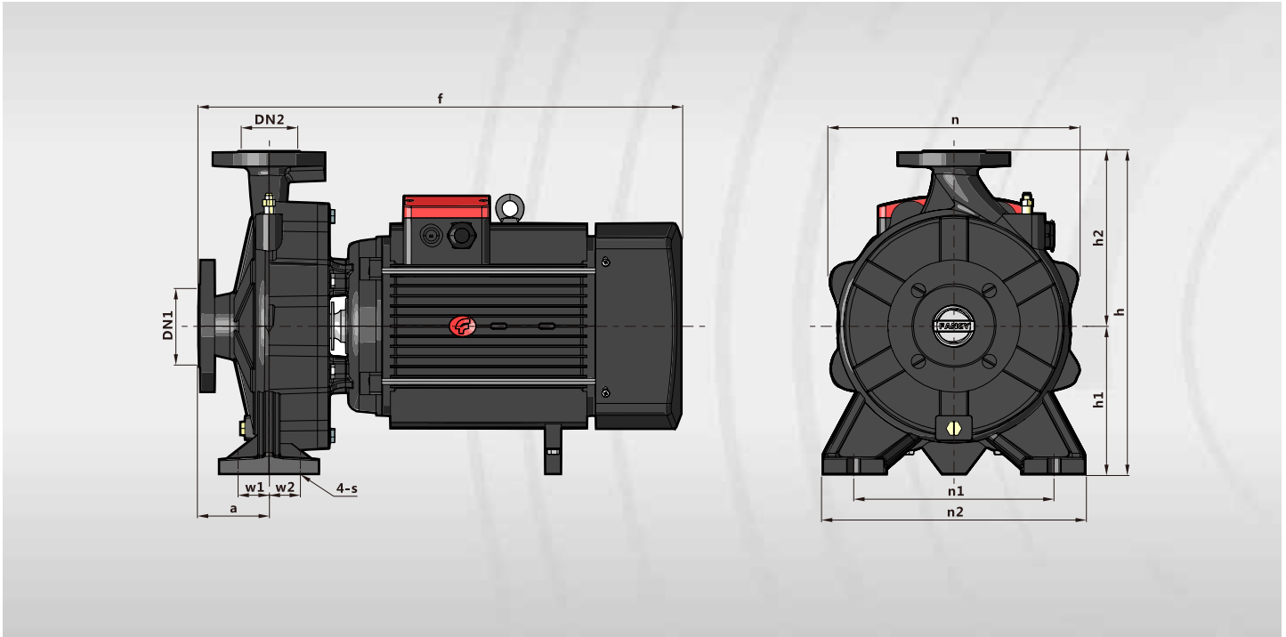
DIMENSIONS AND N.W/DIMENSIONES Y PESOS/DIMENSIONS ET POIDS
