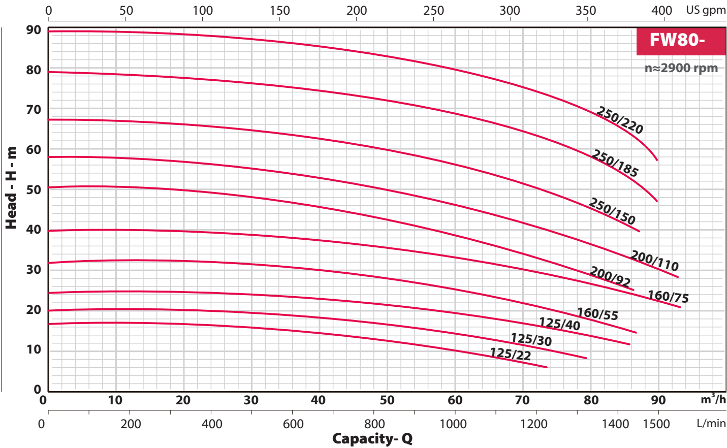
PERFORMANCE CURVE/CURVA DE RENDIMIENTO/COURBE DE PERFORMANCE
